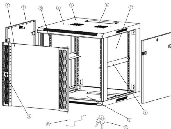
Ilustración de estructura de ensamble
